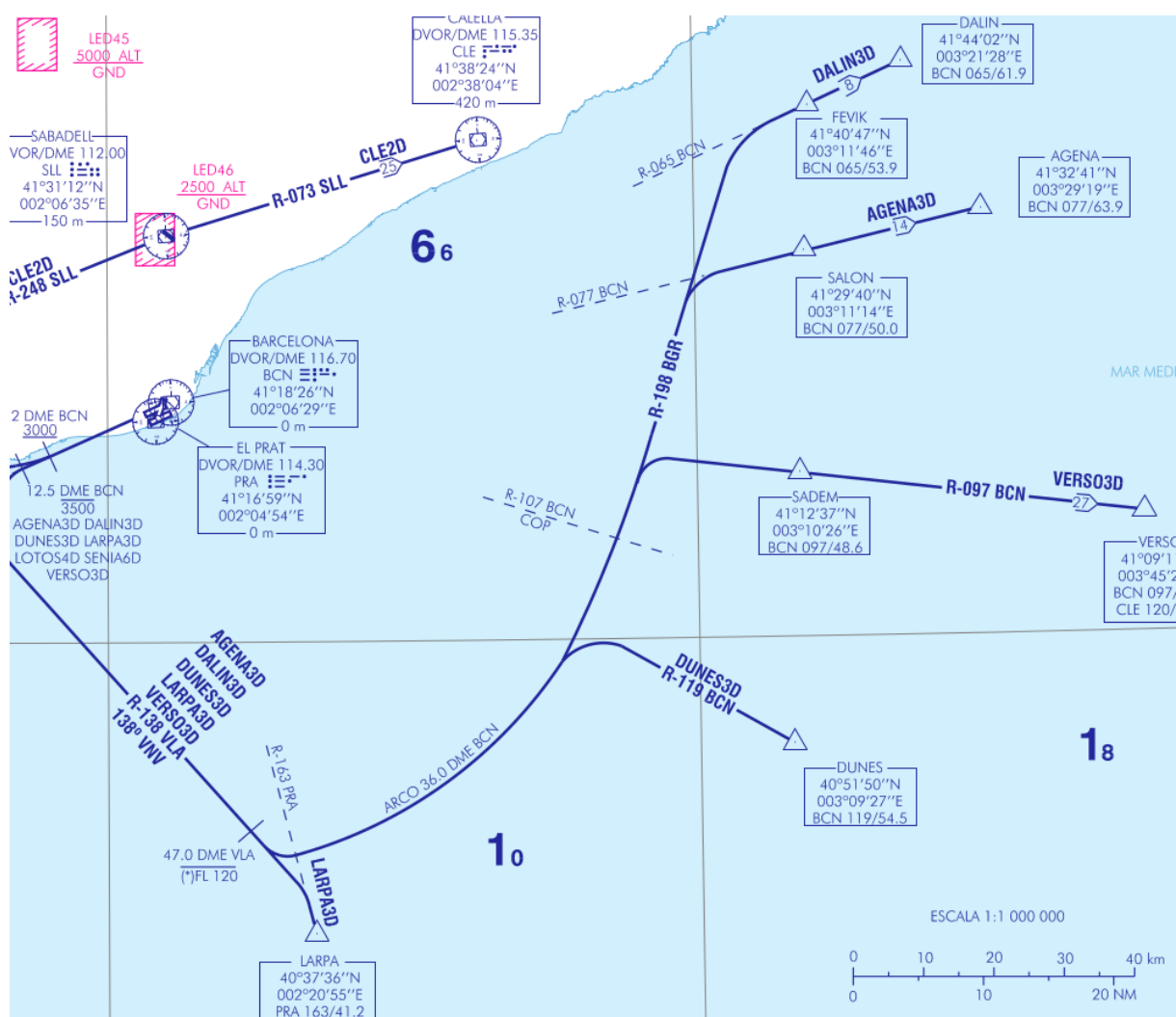
Figura 3.23: Extracto de SID convencional de la RWY 25R de LEBL [Fig28].
