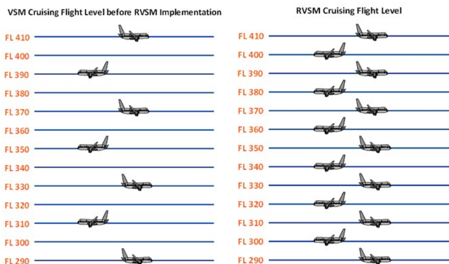
Figura 3.20: Separación Vertical Reducida Mínima, RVSM [Fig24].
